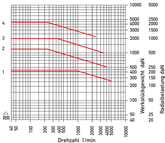
Radial – Typ LRS, LRS G
