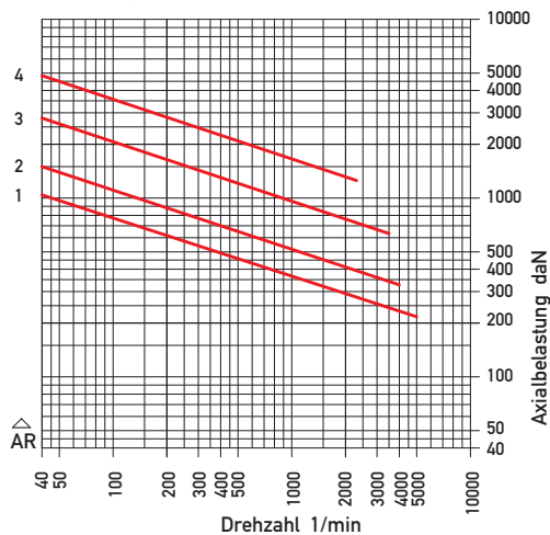
Axial – Typ LRS, LRS G
