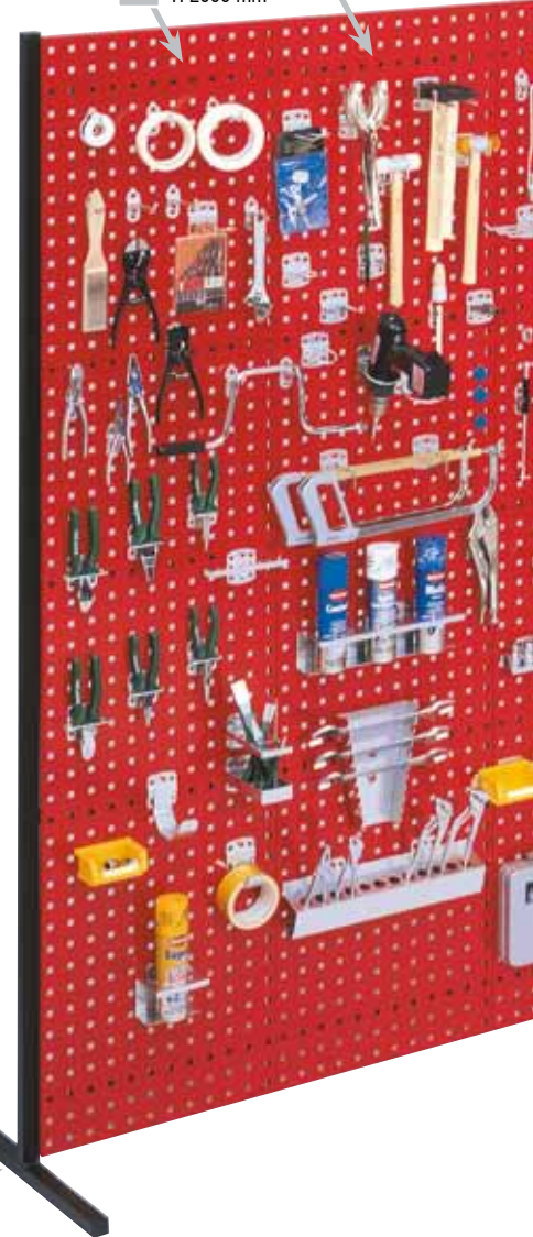
9 Lochplatte H 2000 mm 7 Querverbinder B 1500 mm
